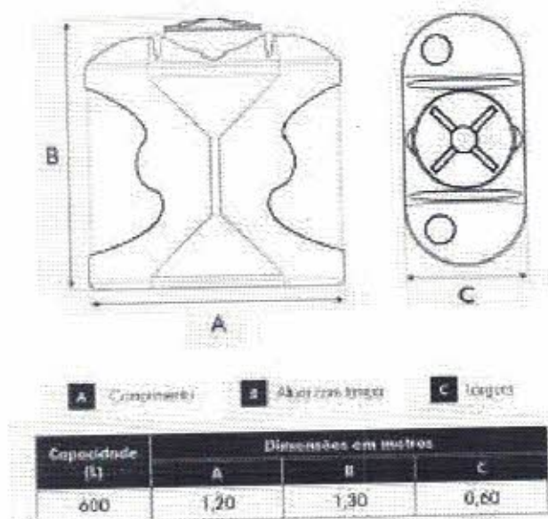
Figura 21 – imagem exemplificativa de croqui da cisterna vertical modular.
